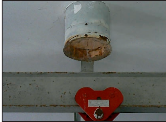
Wskutek wysokiego stężenia siarkowodoru w powietrzu wentylatory w budynku krat gęstych ulegają b. szybkiej korozji
